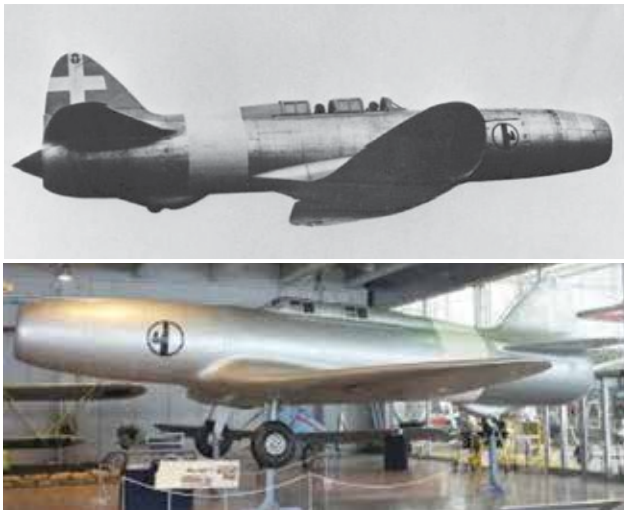
Sopra il prototipo Caproni-Campini (CC2) in volo. In basso il CC2, fortunatamente sfuggito alla distruzione, attualmente presso il Museo dell'Aeronautica di Vigna di Valle
